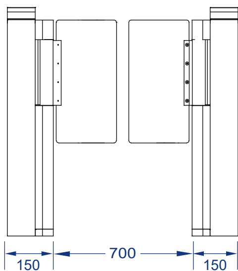
正视图
