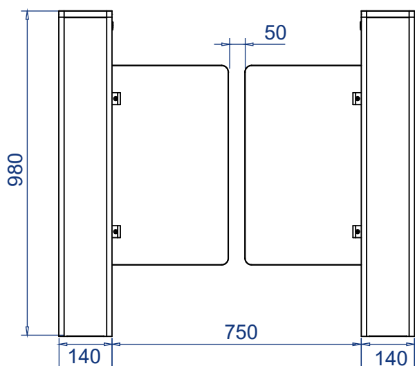
正视图
