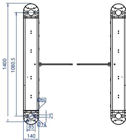
安装底座图
